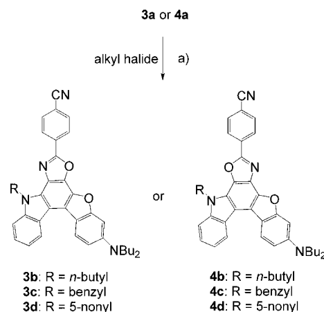
Scheme 2. Synthesis of fluorophores 3 and 4 . a) 3b : iodobutane, NaH, acetonitrile, r.t., 5 h, 82%; 3c : benzyl bromide, NaH, acetonitrile, r.t., 10 h, 79%; 3d : 5-bromononane, NaH, acetonitrile, r.t., 24 h, 74%; 4b : iodobutane, NaH, acetonitrile, r.t., 2 h, 89%; 4c : benzyl bromide, NaH, acetonitrile, r.t., 2 h, 82%; 4d : 5-bromononane, NaH, acetonitrile, r.t., 12 h, 70%.
